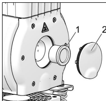
Obr. 13: Výměna vstupního filtru
