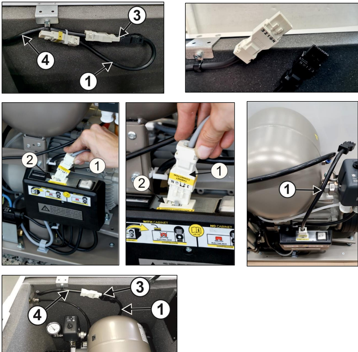
Obr. 8: Připojení skříňky DK50-10S/M ke kompresoru
