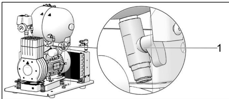
Rys. 11: Spust kondensatu
