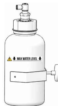
Obr. 10: Kontrola nádoby na sběr kondenzátu
