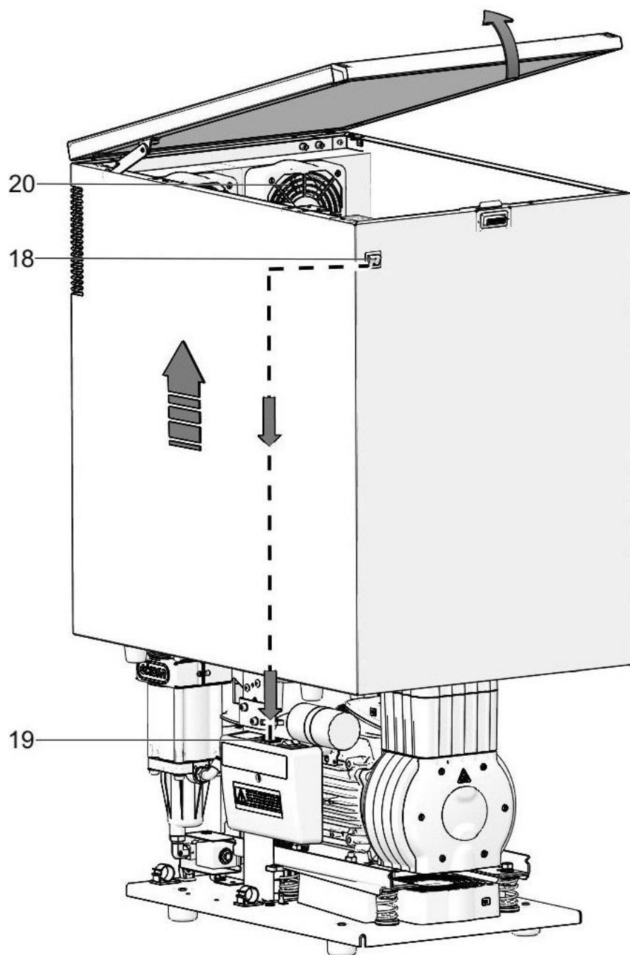
Рис. 3: Шкаф 8-10 bar
