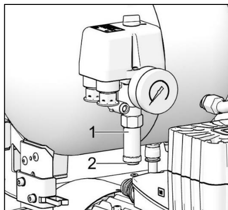
Fig. 12: Contrôle de la soupape de sécurité
