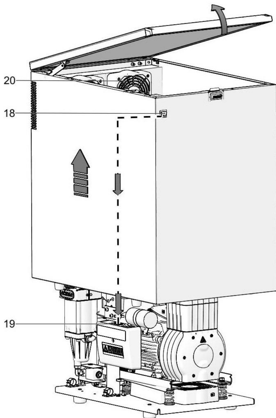
Obr. 3: Skříňka 8-10 bar
