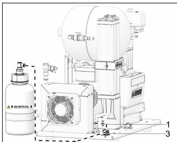
Рис. 7: Слив конденсата
