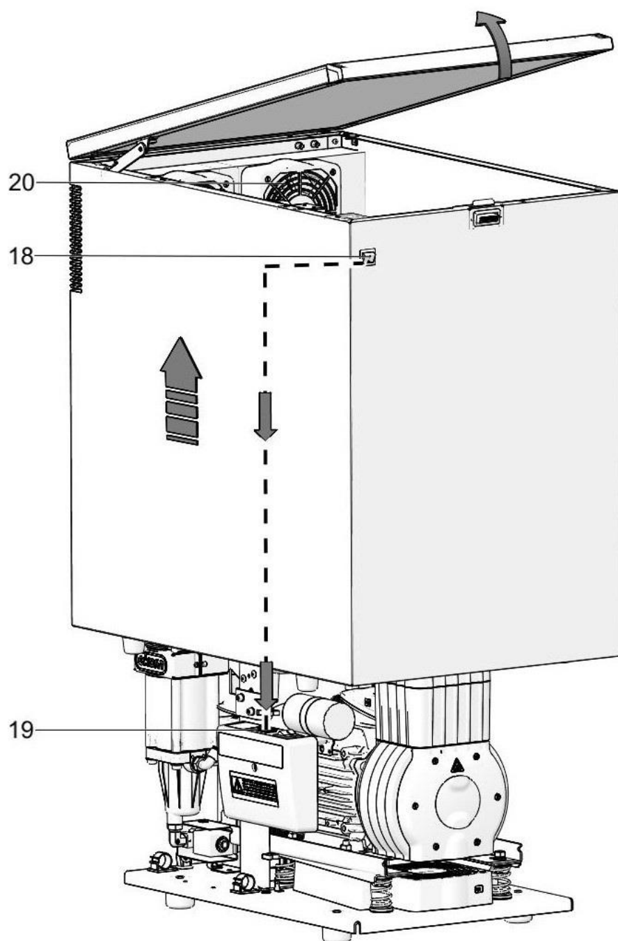
Obr. 3: Skrinka 8-10 bar
