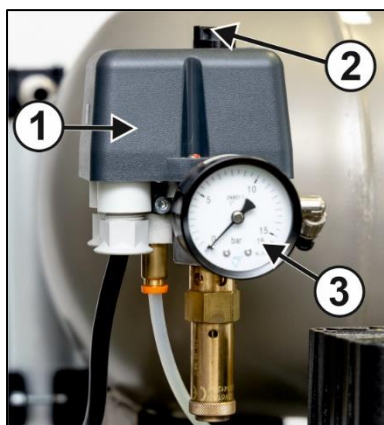
Rys. 9: Włączanie sprężarki
