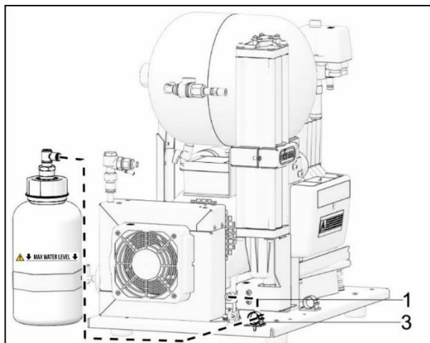
Obr. 7: Výstup kondenzátu
