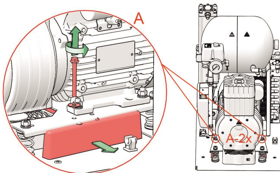
Obr. 5: Odjištění agregátu
