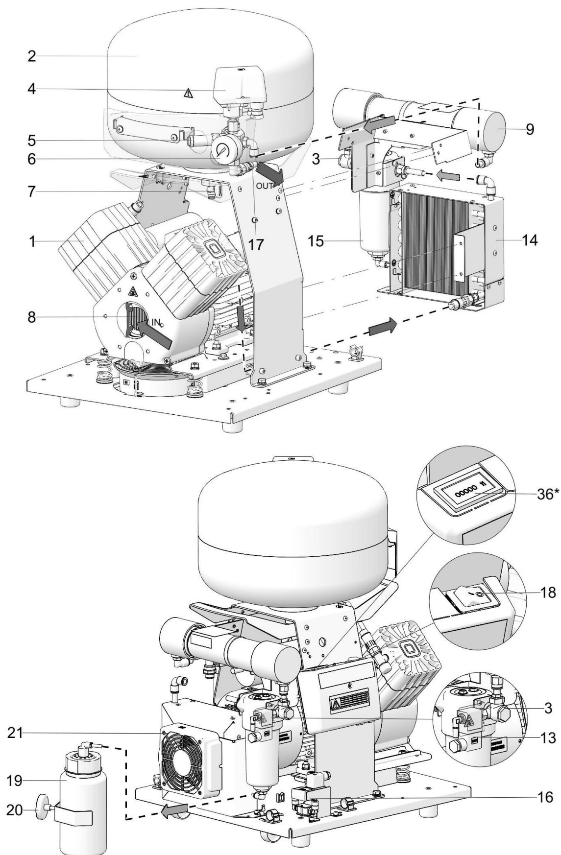
Fig. 2 - DK50 2V/M - Compresseur avec sécheur
