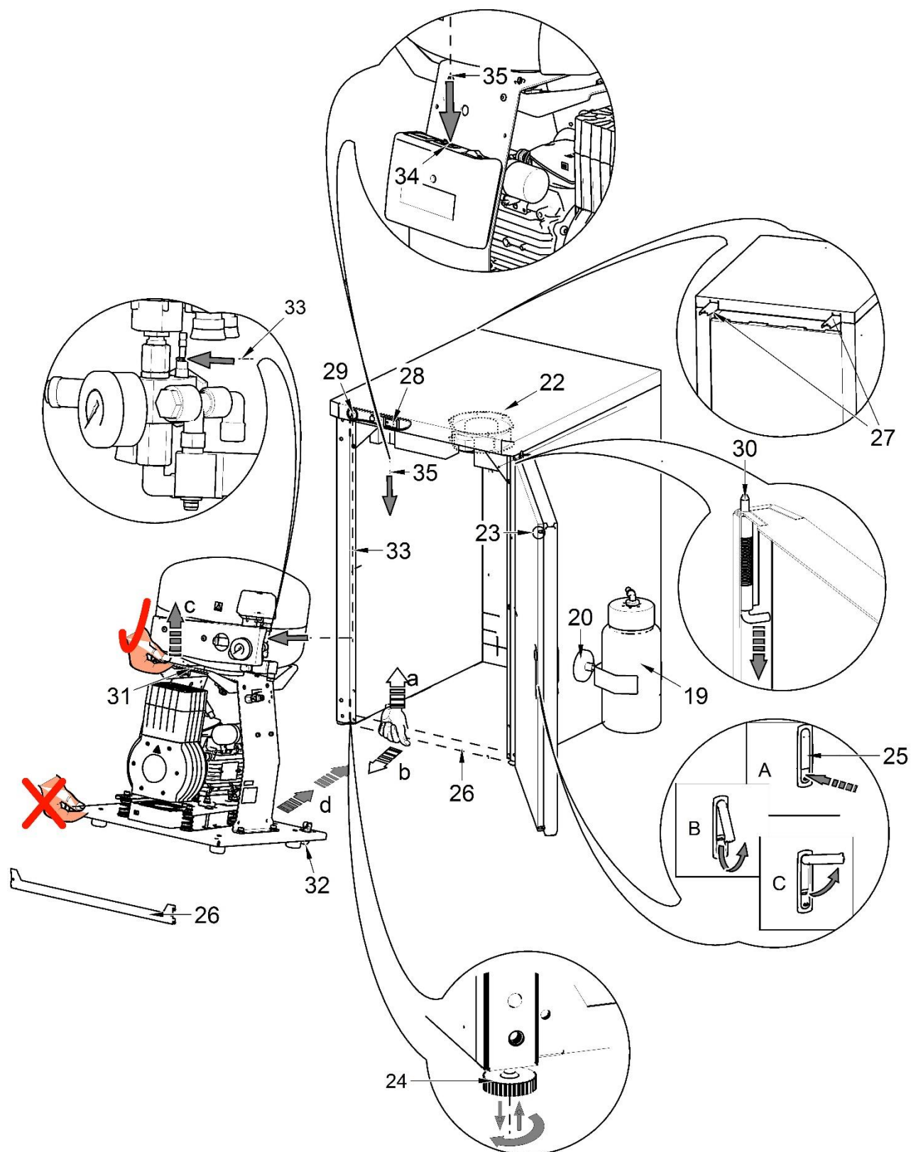
Рис. 3. - Шкаф
