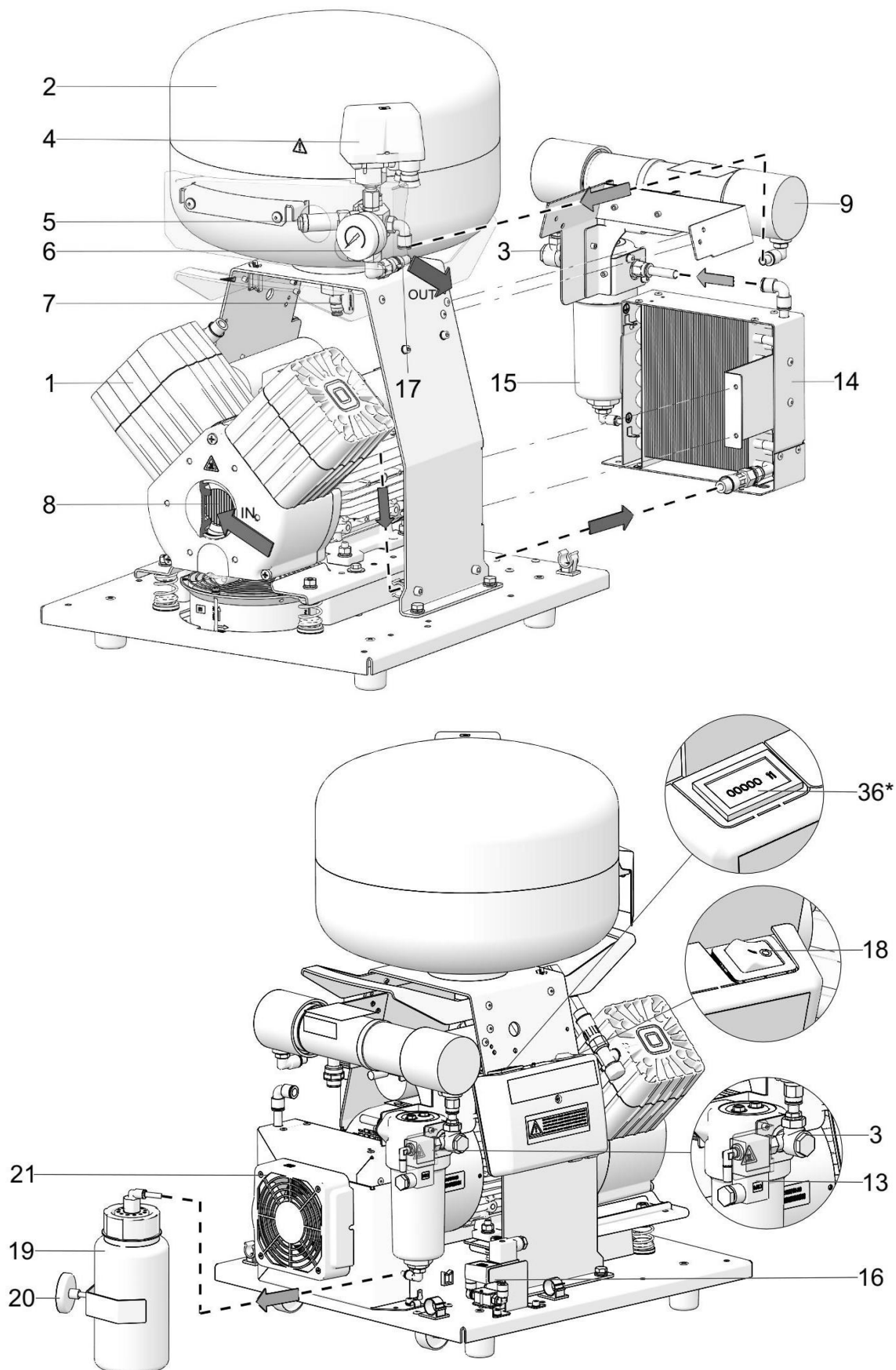
Rys. 2 – DK50 2V/M – sprężarka z osuszaczem
