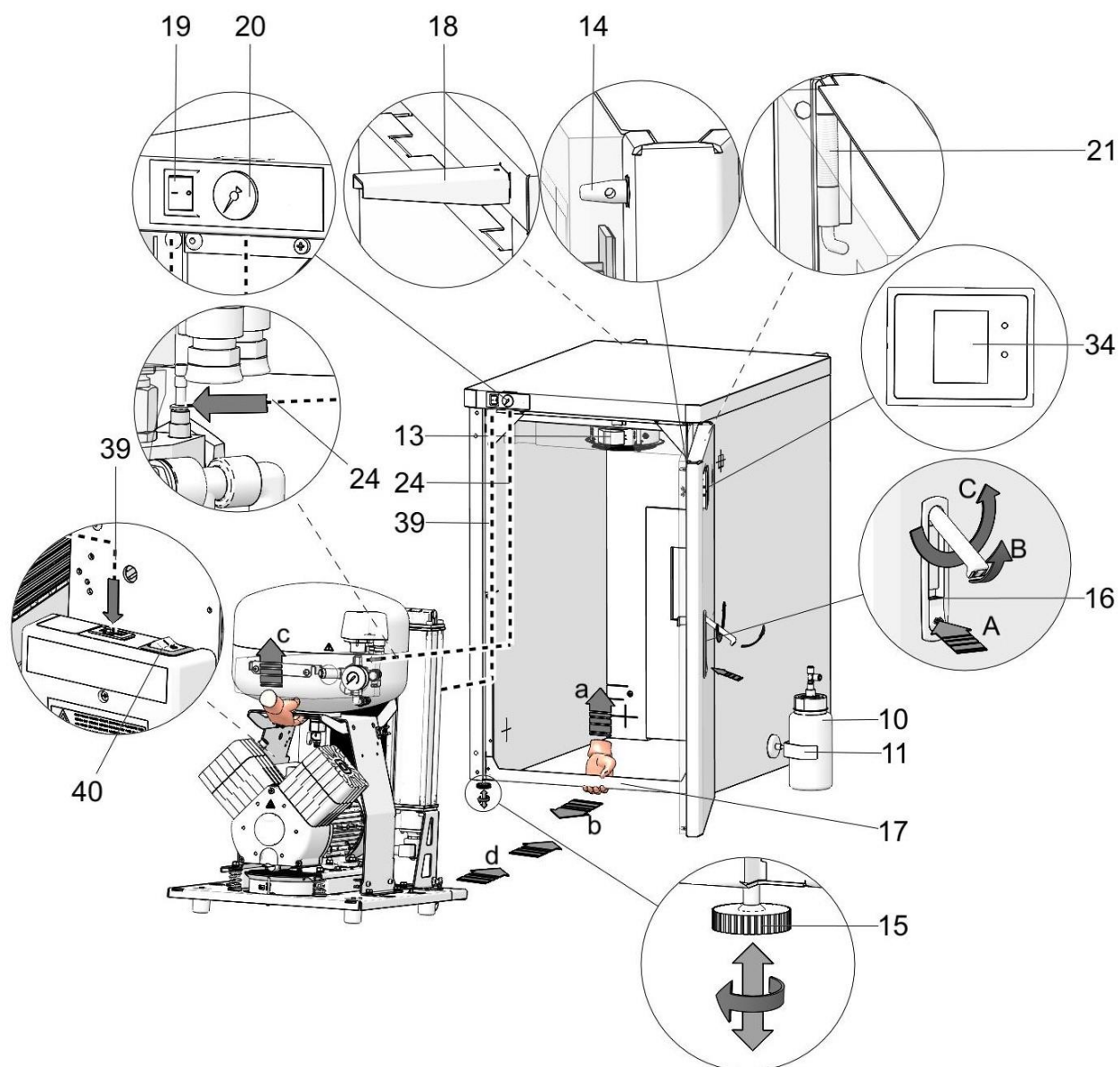
Рис. 3: – Шкаф
