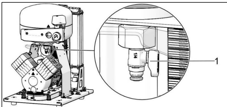
Fig. 19: Purge de condensat
