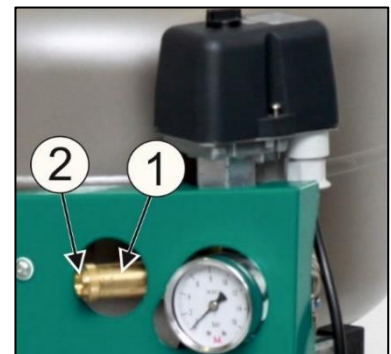
Abb. 20: Sicherheitsventil überprüfen
