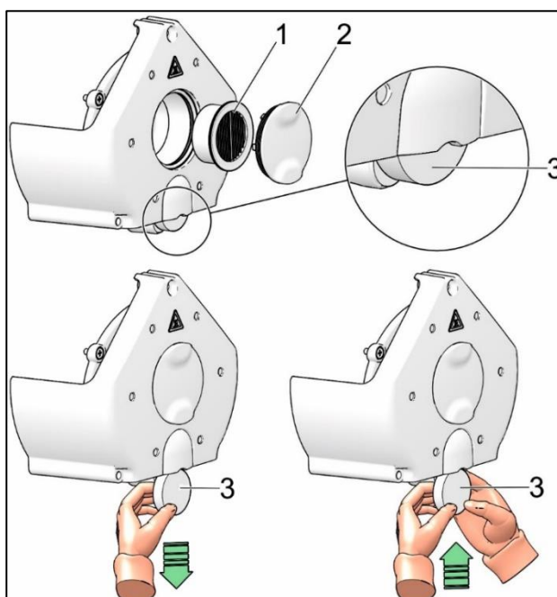
Obr. 21: Výmena vstupného filtra
