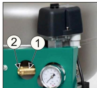
Rys. 20: Kontrola zaworu bezpieczeństwa
