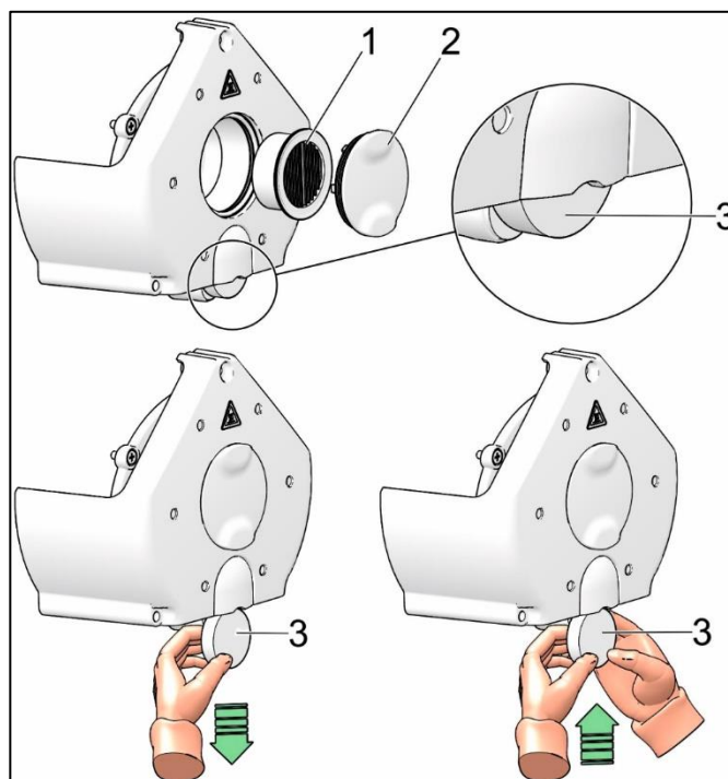
Rys. 21: Wymiana filtra wlotowego i wstępnego
