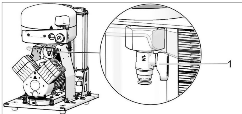
Рис. 19: Слив конденсата
