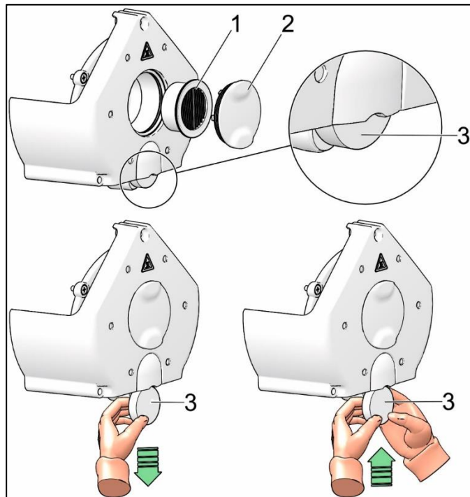
Abb. 21: Austausch des Ansaugfilters und Vorfilters
