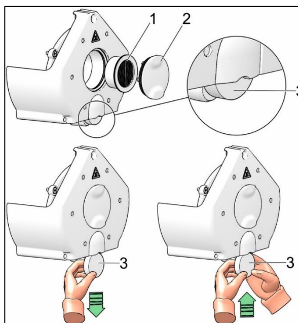
Fig. 21: Remplacement du filtre d'entrée
