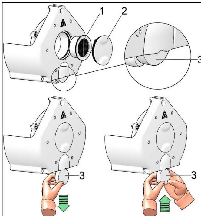
Рис. 21: Замена входного фильтра и фильтра предварительной очистки
