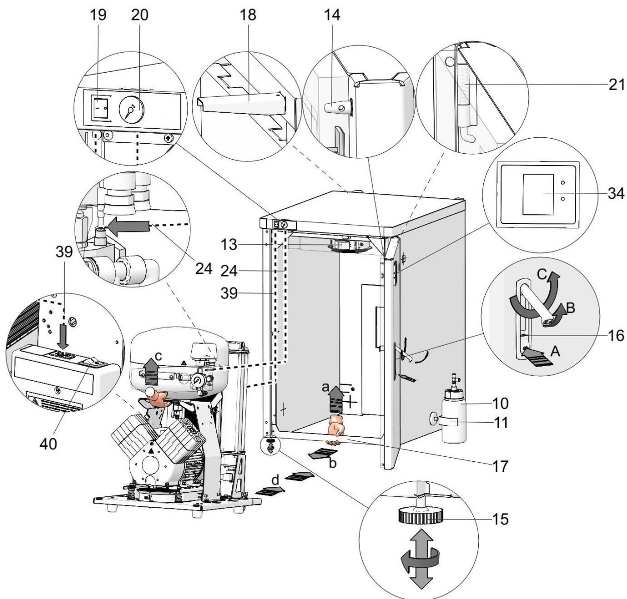
Fig. 3: – Armoire
