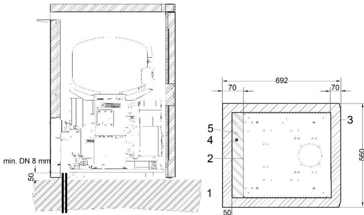
Rys. 9: Instalacja podłogowa
