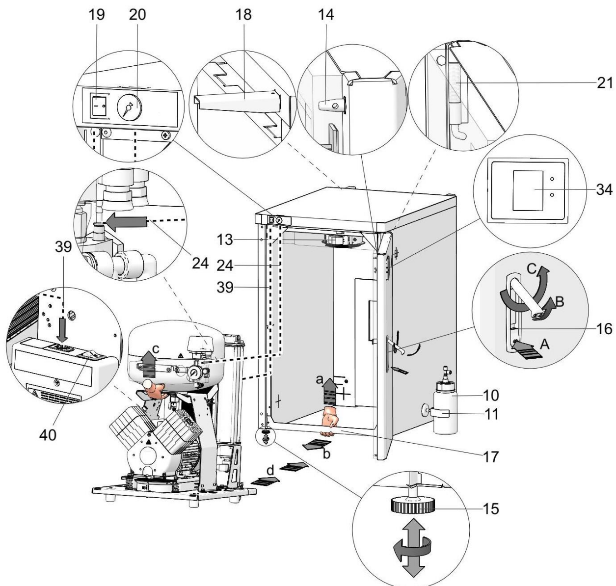
Obr. 3: – Skrinka
