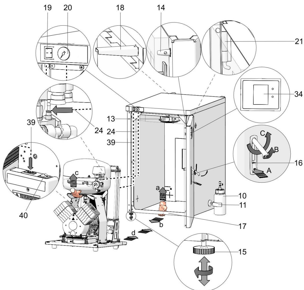
Rys. 3: – Obudowa
