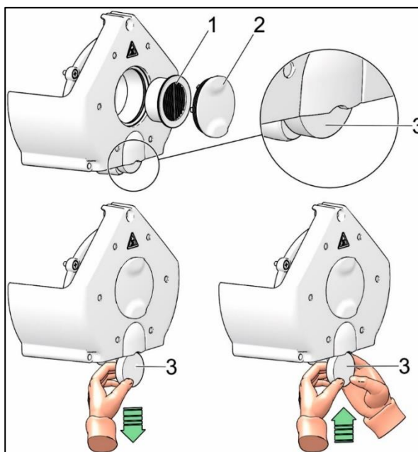
Obr. 21: Výměna vstupního filtru a předfiltru
