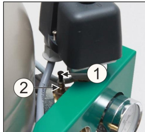
Abb. 7: Verbinden des Gehäuse-Druckmessers mit dem Kompressor
