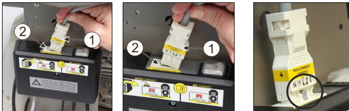
Fig. 11: Raccordement de l'armoire au compresseur
